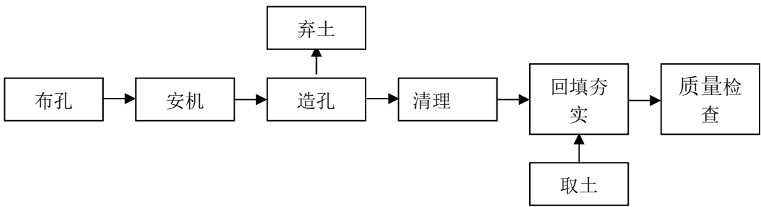
图 2-1 套井冲抓回填施工工艺流程图
