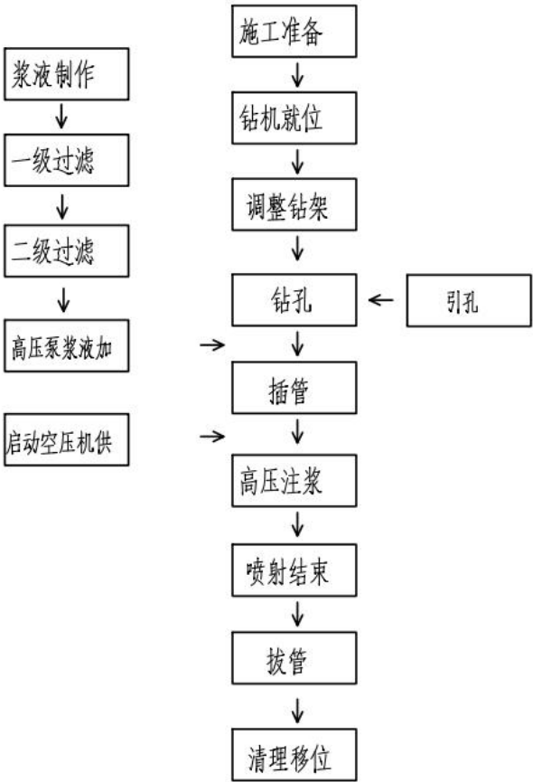
图 2-2 高喷灌浆施工工艺流程
